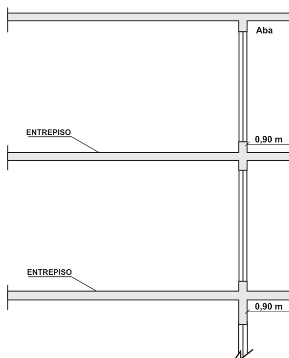
Figura A3 - Modelo de compartimentação vertical (abas)
