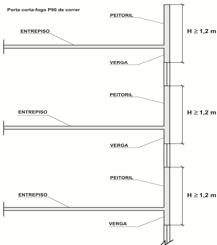
Figura A2 - Modelo de compartimentação vertical (verga-peitoril)
