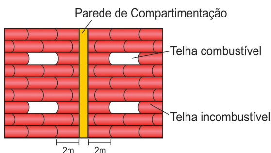
Figura 1 – Afastamento de telhas combustíveis
